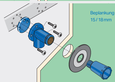
Armaturenanschlusswinkel 1/2" x 1/2" erfüllt ÖNORM B 3407 und Trinkwassertauglichkeit mit ÜA-Kennzeichnung
