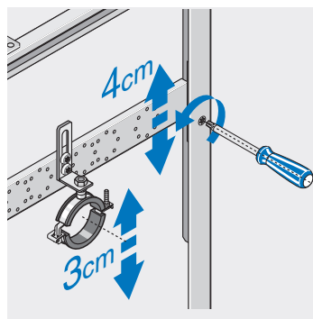
höhenverstellbare Armaturenanschlussplatte mit separat verstellbarer Rohrschelle
