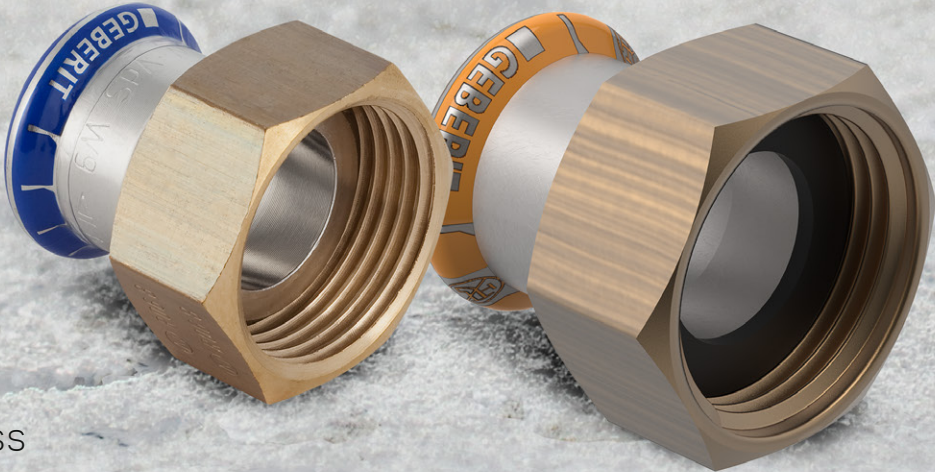
Geberit Mapress Edelstahl und Mapress Therm Übergang mit Überwurfmutter
