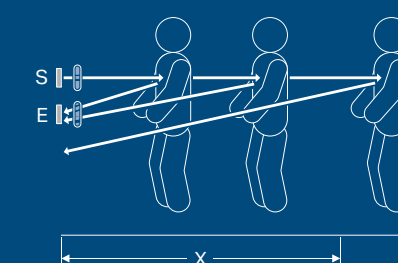
↑ Zuverlässige Nutzererkennung im Distanzbereich 100 – 600 mm.
