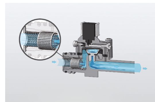
↑ Innovatives Filtersystem für hohe Funktionssicherheit.
