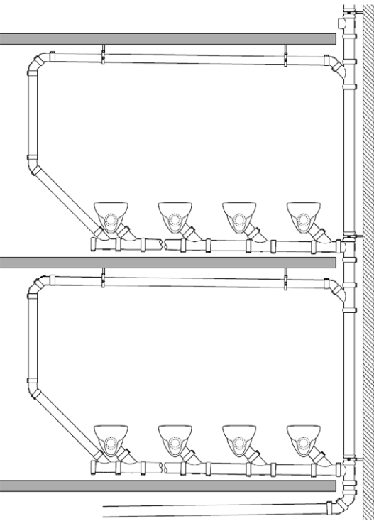
Sammelanschlussleitung mit Umlüftung
