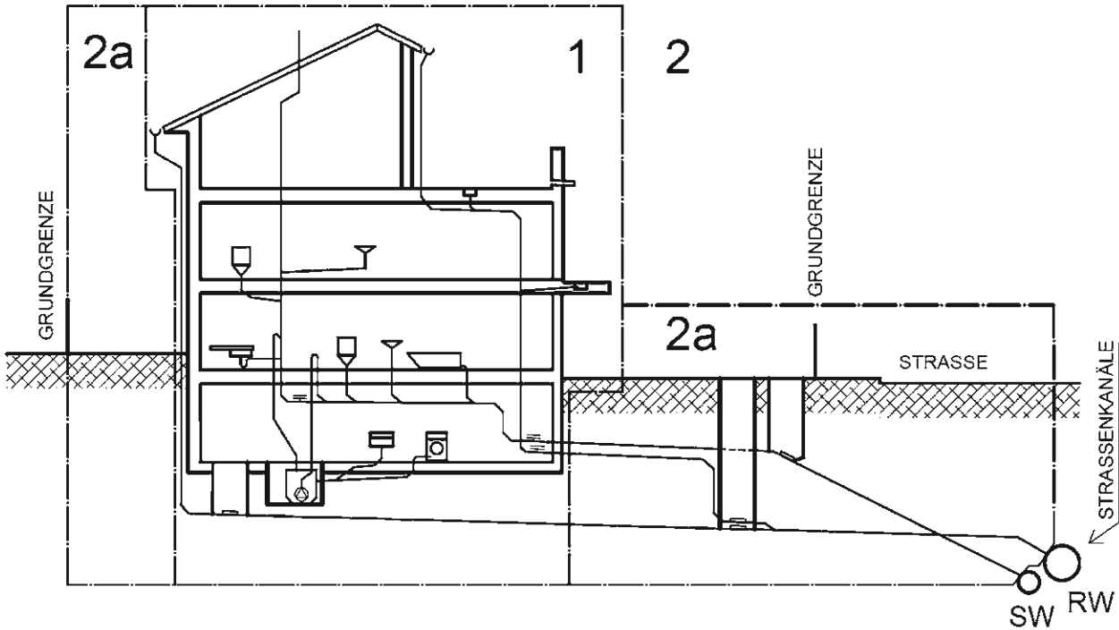
Prinzipskizze Anwendungsbereich
