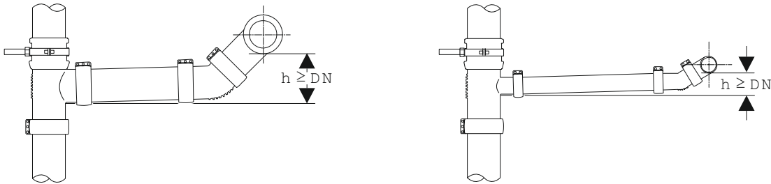
Einmündung von Anschlussleitungen in eine Fallleitung
