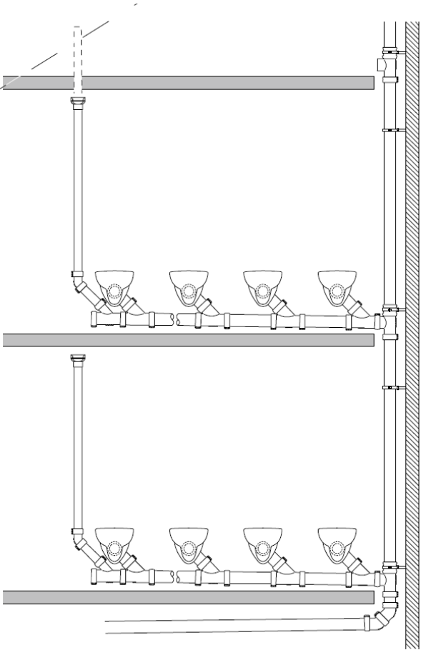
Belüftungsventil als Ersatz für eine Umlüftung oder eine indirekte Nebenlüftung.
