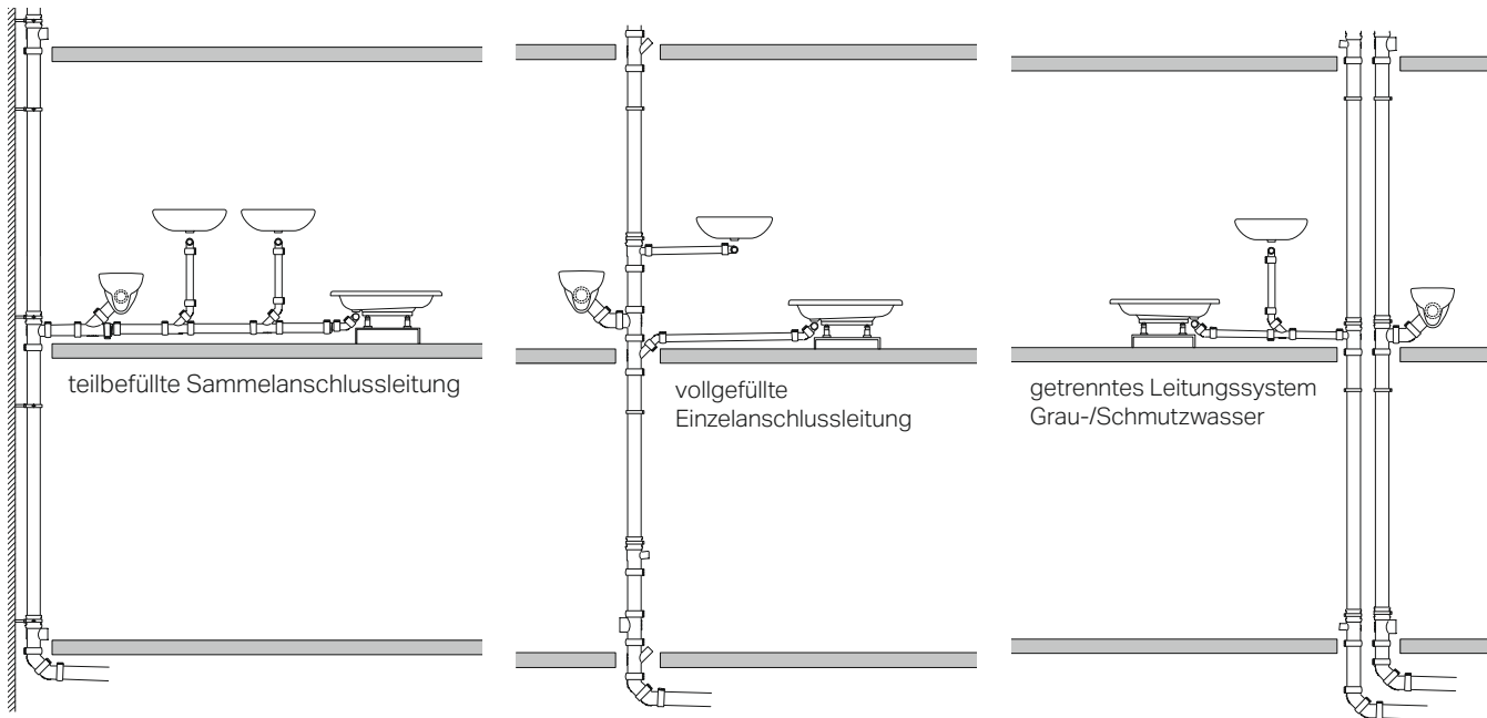
Entwässerungsanlage System I und II: In Österreich ist System I anzuwenden (Füllungsgrad 0,5). System II mit Füllungsgrad 0,7. Entwässerungsanlage System III Entwässerungsanlage System IV
