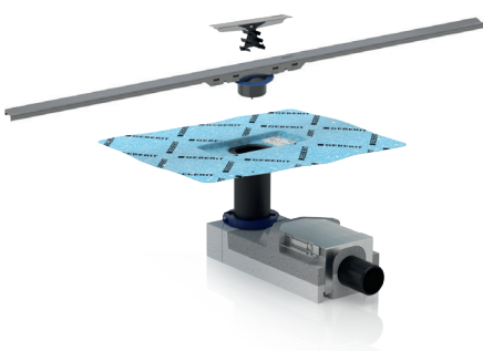
Rohbauset für Duschrinne CleanLine Einbauhöhe ab 90 mm: 154.150.00.1 Einbauhöhe ab 65 mm: 154.152.00.1 Duschrinne CleanLine50 Abbildung Art.Nr.: 154.446.QC.1
