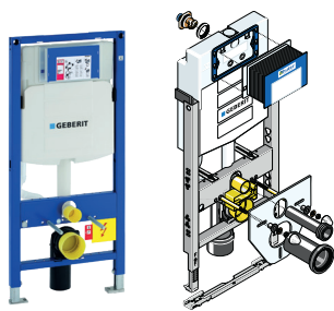
WC-Element Geberit Duofix 111.921.00.x oder Huter HU-WC 1025-E
