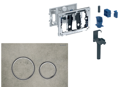
Betätigungsplatte Sigma50 round mit Einschub für DuoFresh Stick Abbildung Art.Nr.: 115.884.JV.1 und 115.062.21.1
