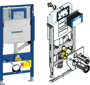
WC-Element mit externem Geruchsabsauganschluss Geberit Duofix 111.367.00.x oder Huter HU-WC 1023-G
