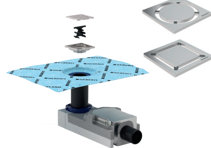
Bodenablauf für Dusche Einbauhöhe ab 90 mm: 154.050.00.1 Einbauhöhe ab 65 mm: 154.052.00.1 Designrost Circle Abbildung Art.: 154.311.00.1 Designrost Square Abbildung Art.: 154.312.00.1
