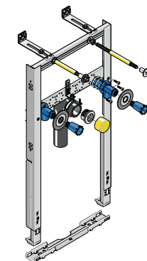
Waschtisch-Element Geberit Duofix WT 111.436.00.x (Abb. siehe oben) oder Huter HU-WT 2010-M
