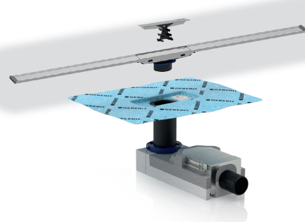
Rohbauset für Duschrinne CleanLine Einbauhöhe ab 90 mm: 154.150.00.1 Einbauhöhe ab 65 mm: 154.152.00.1 Duschrinne CleanLine 20 Abbildung Art.Nr.: 154.450.KS.1
