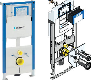
WC-Element Geberit Duofix 111.311.00.x oder Huter HU-WC 1020-G
